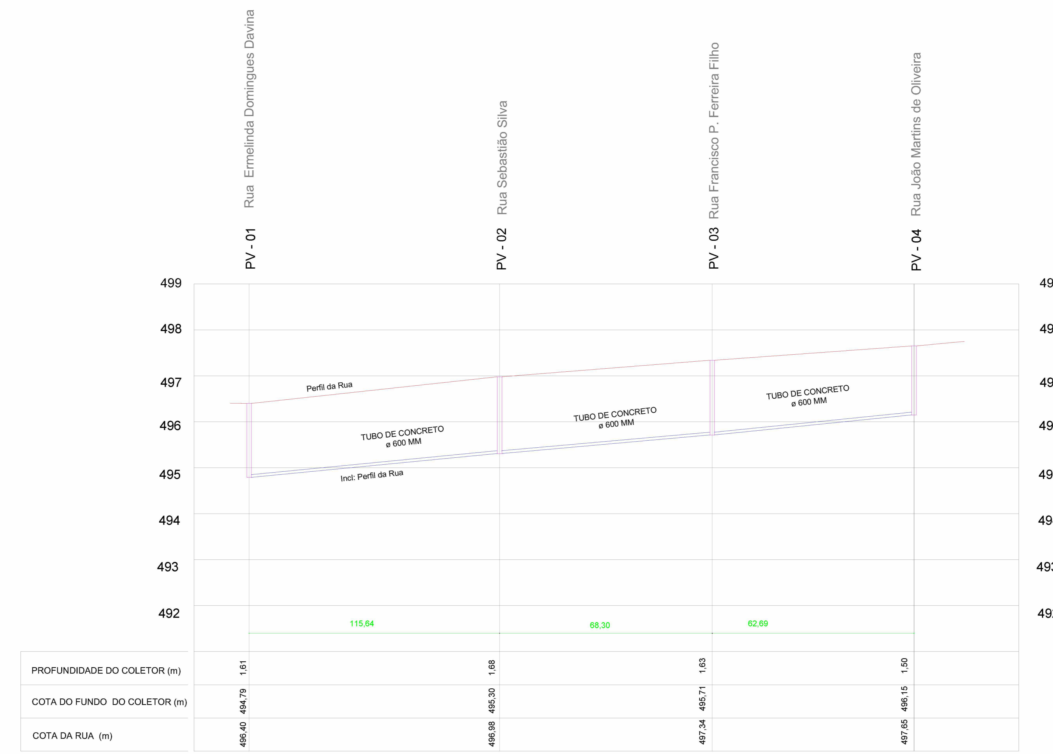
PERFIL LONGITUDINAL TRECHO-03 RUA EDUARDO MARTINS ROMEIRA ESC. HORIZONTAL = 1 : 1000 ESC. VERTICAL = 1 : 100
