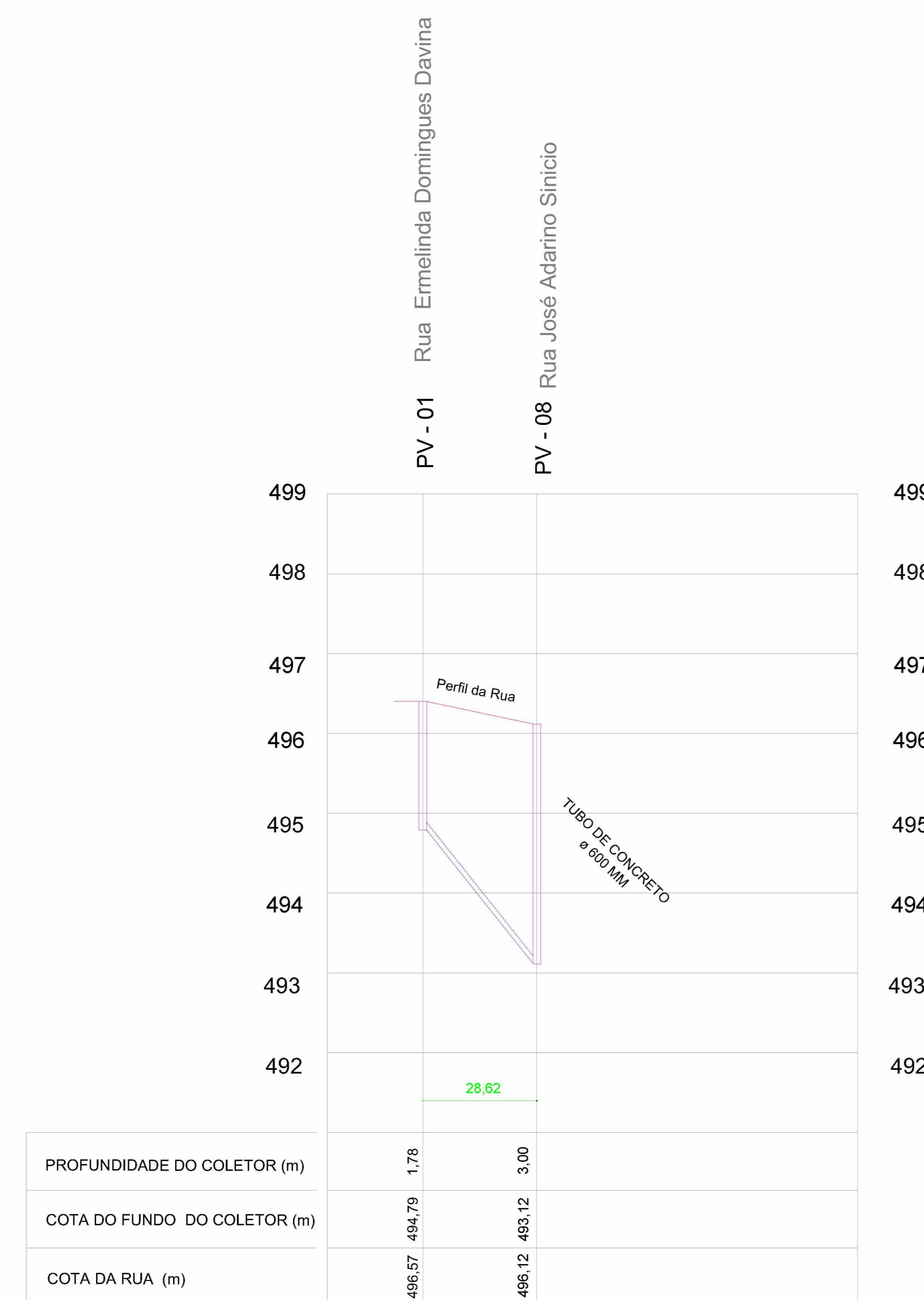
PERFIL LONGITUDINAL TRECHO-03 RUA ERMELINDA DOMINGUES DAVINA ESC. HORIZONTAL = 1 : 1000 ESC. VERTICAL = 1 : 100
