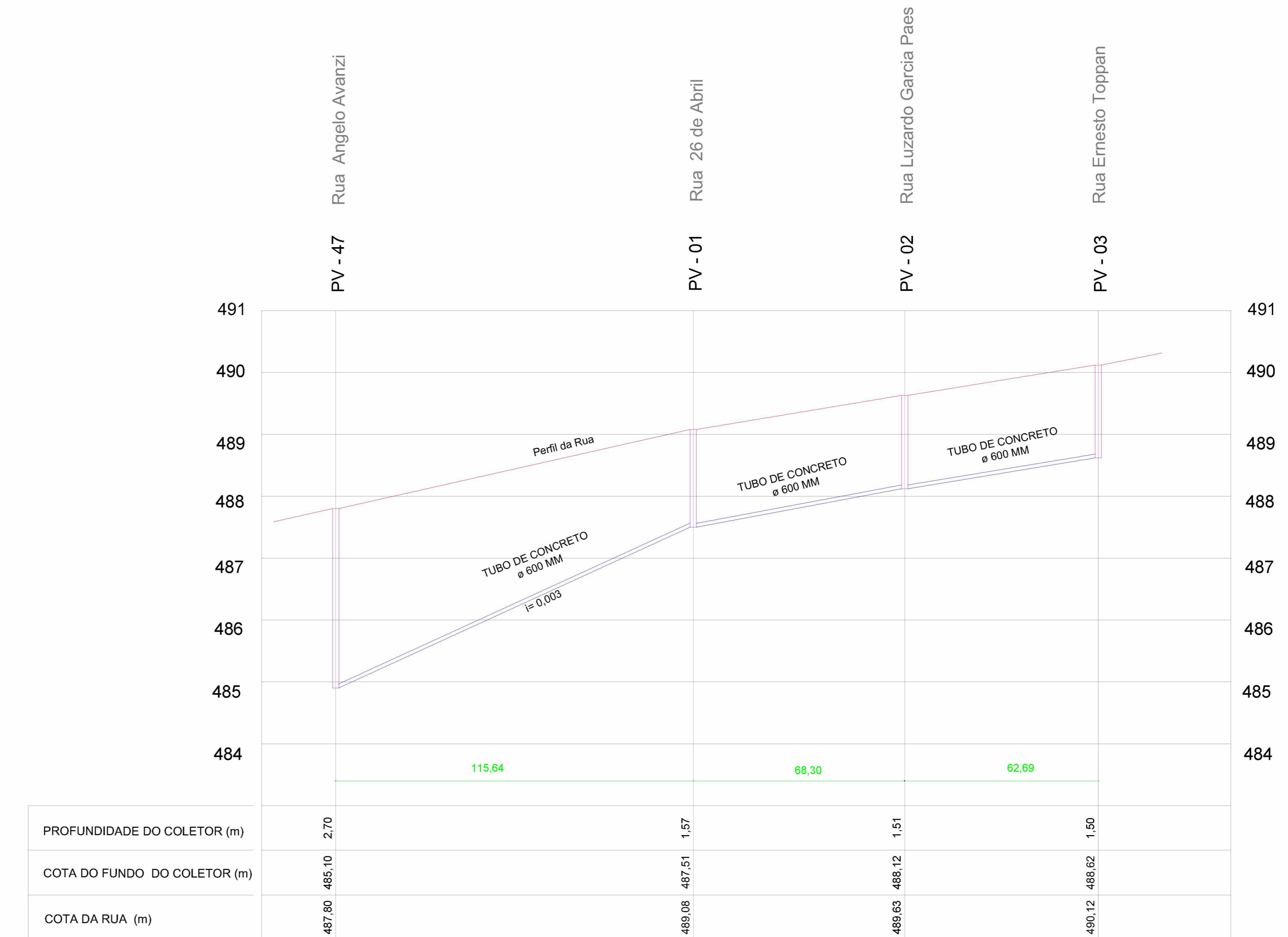
PERFIL LONGITUDINAL TRECHO-02 RUA ANTONIO LUIZ VIANA ESC. HORIZONTAL = 1 : 1000 ESC. VERTICAL = 1 : 100
