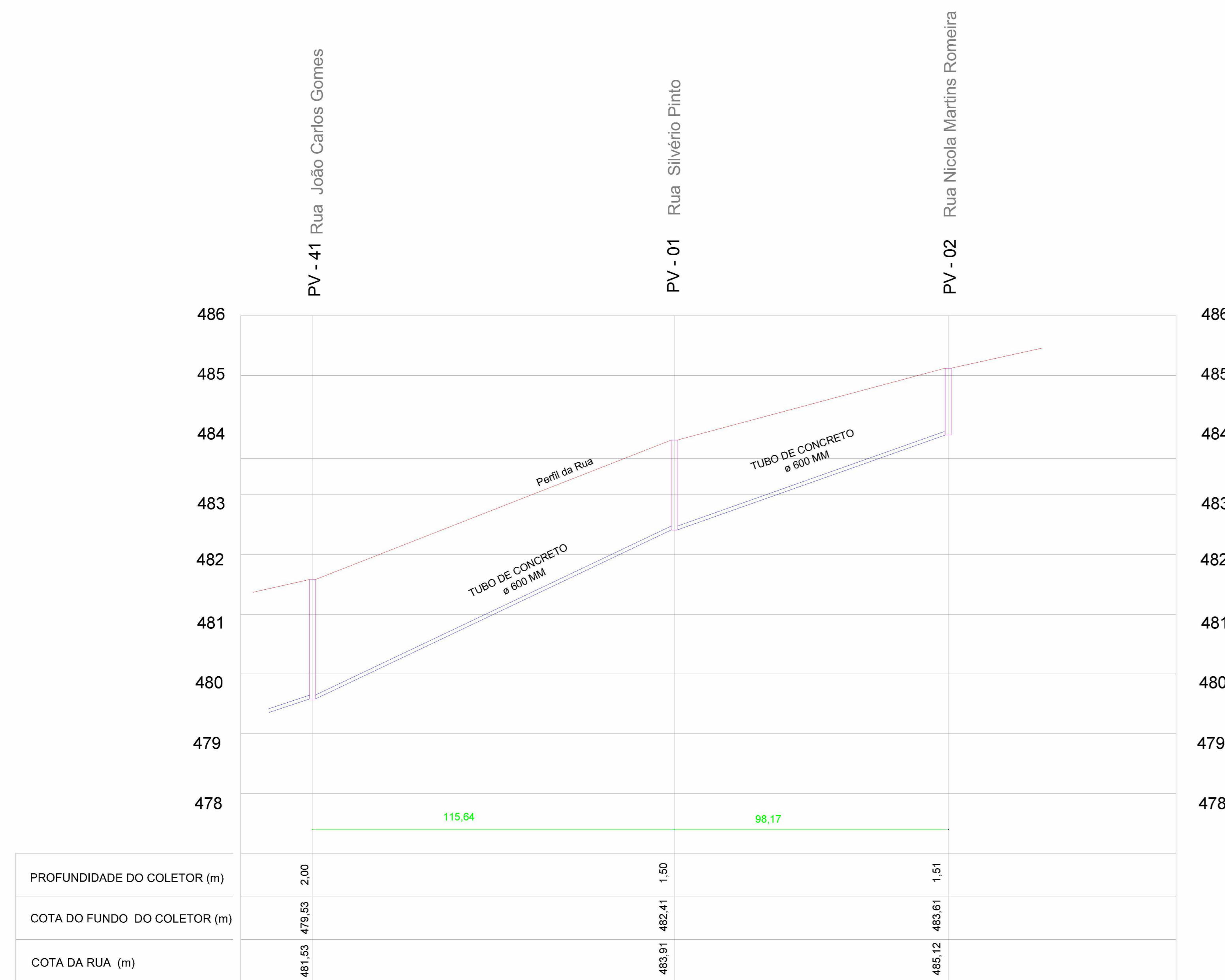
PERFIL LONGITUDINAL TRECHO-01 RUA TIRADENTES ESC. HORIZONTAL = 1 : 1000 ESC. VERTICAL = 1 : 100
