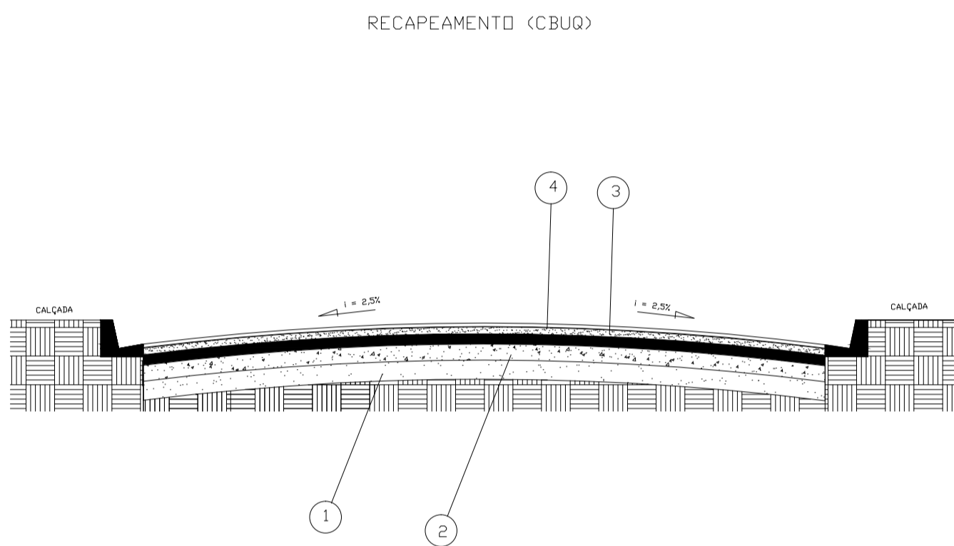
SEÇÃO TIPO DO PAVIMENTO S/ESCALA
