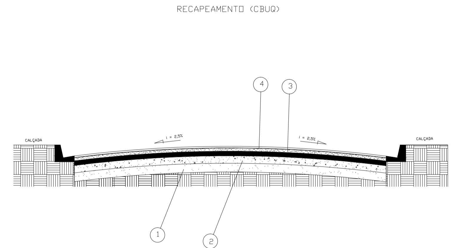
SEÇÃO TIPO DO PAVIMENTO S/ESCALA
