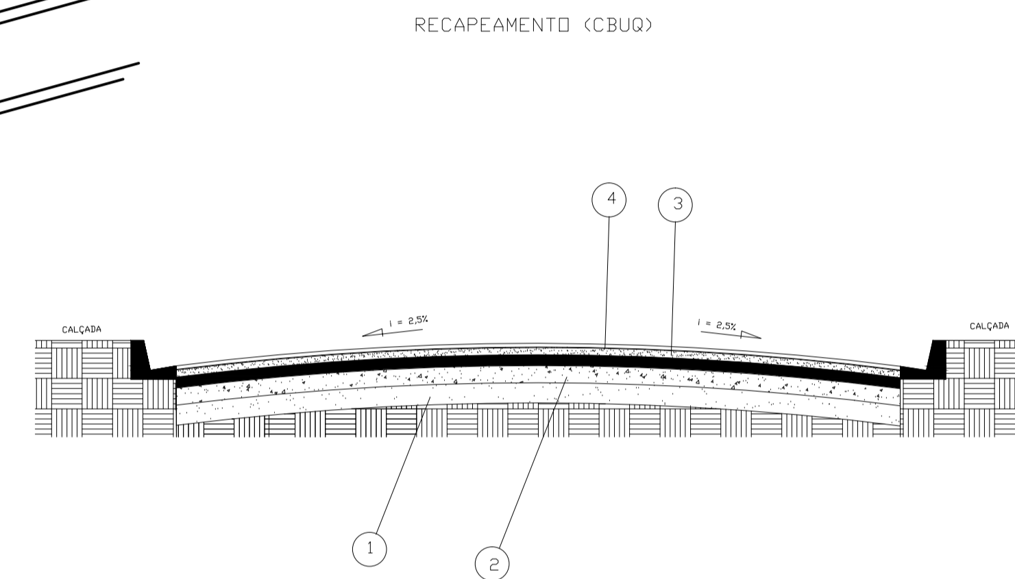
SEÇÃO TIPO DO PAVIMENTO S/ESCALA
