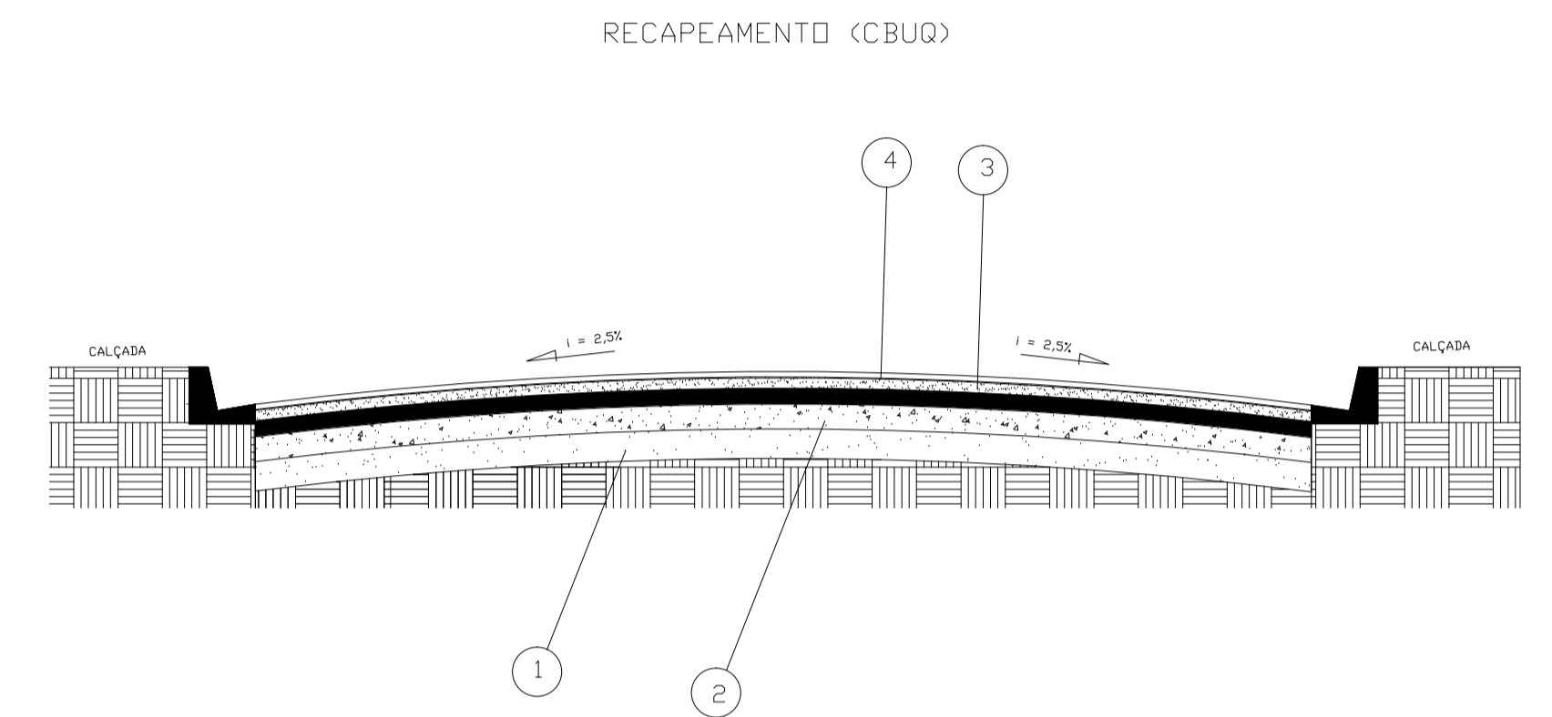
SEÇÃO TIPO DO PAVIMENTO S/ESCALA
