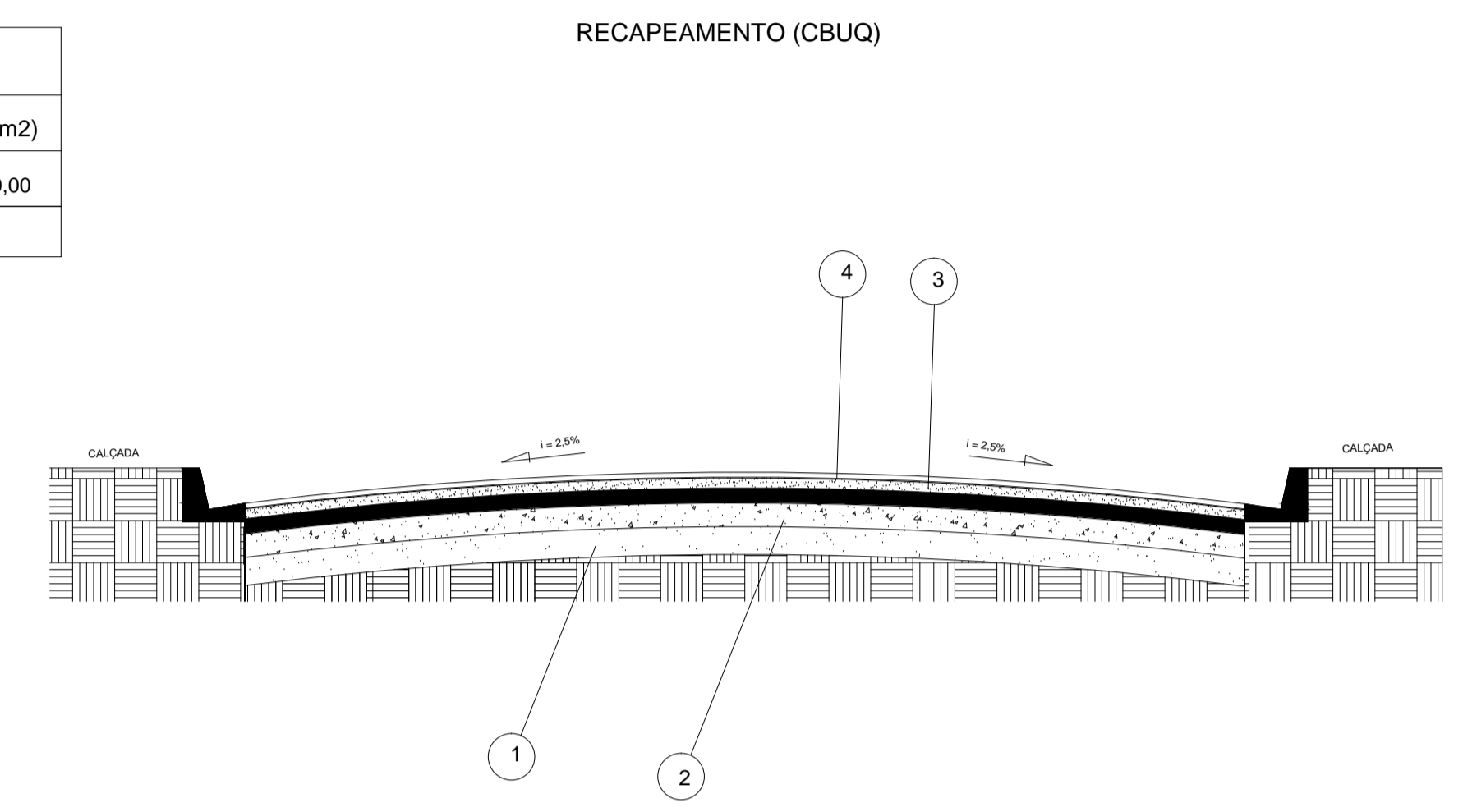
SEÇÃO TIPO DO PAVIMENTO S/ESCALA
