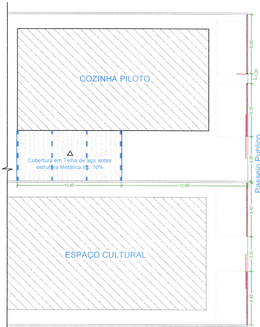
PLANTA BAIXA ESC. 1:200
