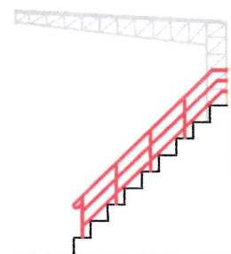
Detalhe Guarda-Corpo ESC.: 1:200
