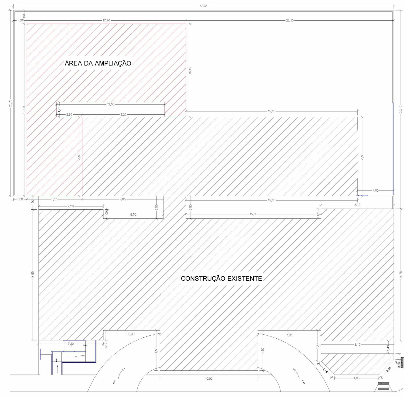
PLANTA DE LOCALIZAÇÃO Esc. 1:200
