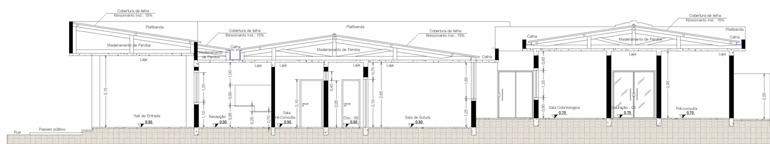
CORTE - GG Escala: 1:100
