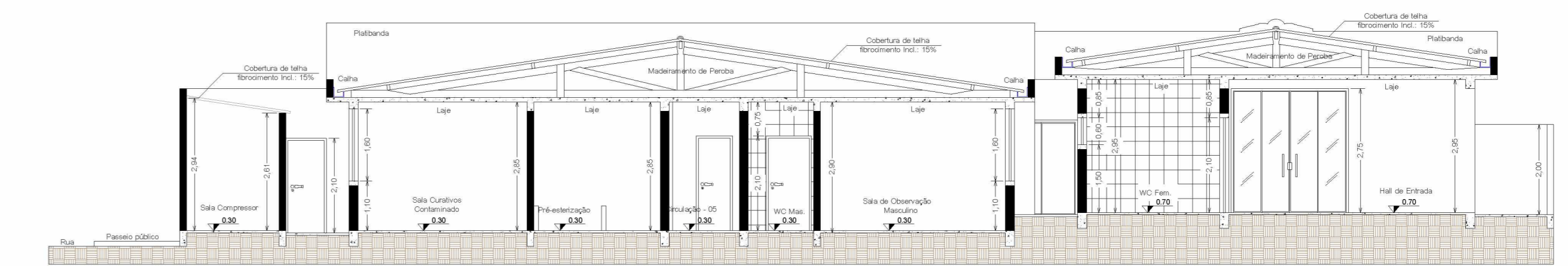
CORTE - FF Escala: 1:100
